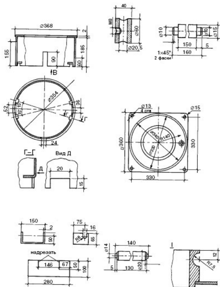
Рис. 101 (продолжение). Конструктивная схема водоподъемника: 1 – кожух приводного механизма; 2 – втулка стойки вала; 3 – пластина стабилизатора; 4 – труба стабилизатора; 5 – основание; 6 – вал; 7 – опорный ролик; 8 – корпус приводного механизма; 9 – приводной ролик; 10 – лента-транспортер; 11 – натяжной механизм; 12 – стяжной валик; 13 – рамка основания; 14 – обойма отжимного устройства; 15 – противовес; 16 – ось обоймы отжимного устройства; 17 – водоприемник; 18 – сливной штуцер; 19 – ось стяжного валика
